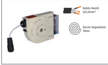
Monofaze - Elektrik Aktarım Tamburu Kilitlemeli - Plastik Gövde
