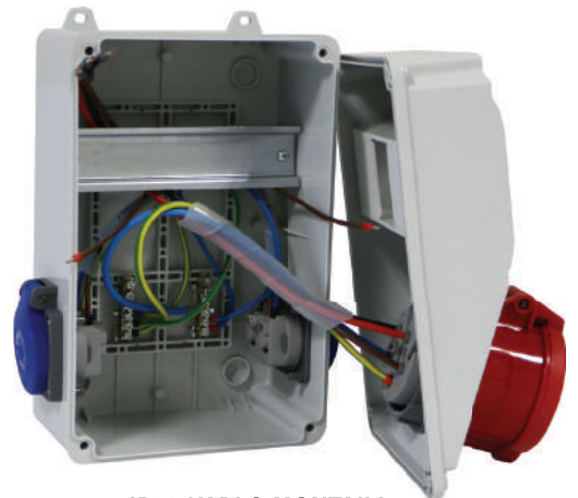
IP44 KABLO MONTAJLI KOMBİNASYON
