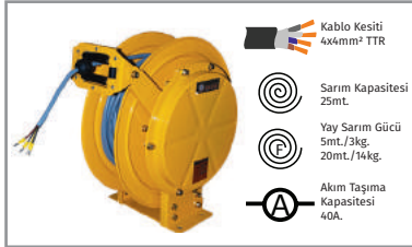
Trifaze - Elektrik Aktarım Tamburu Kilitlemeli - Metal Gövde
