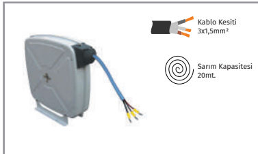
Monofaze - Elektrik Aktarım Tamburu Kilitlemeli - Metal Gövde
