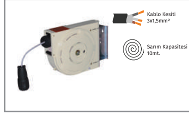
Monofaze - Elektrik Aktarım Tamburu Kilitlemesiz - Plastik Gövde
