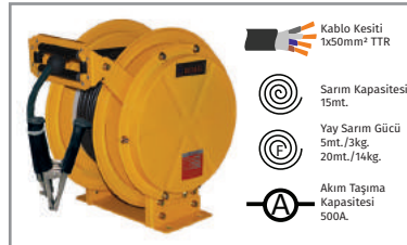
Topraklama ve Kaynak için Elektrik Aktarım Tamburu Kilitlemeli - Metal Gövde
