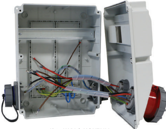
IP67 KABLO MONTAJLI KOMBİNASYON
