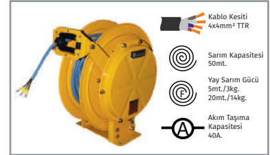
Trifaze - Elektrik Aktarım Tamburu Kilitlemeli - Metal Gövde
